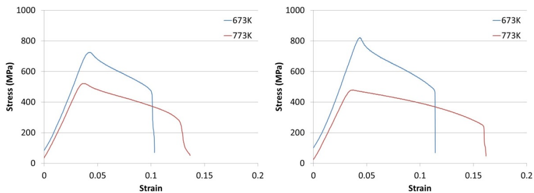
F82H-IEA heat
